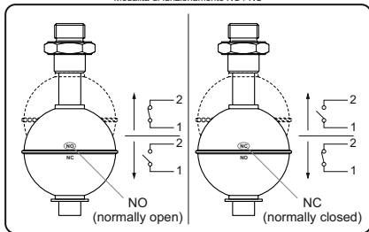
Modalità di funzionamento NO / NC
