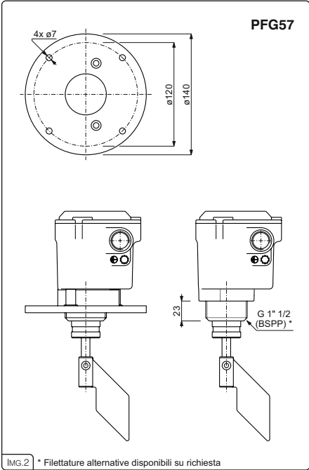
IMG.2 * Filettature alternative disponibili su richiesta
